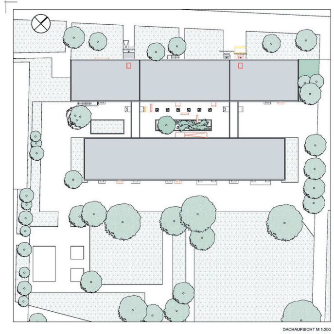
DACHAUFSICHT M 1:200 © Renatus
